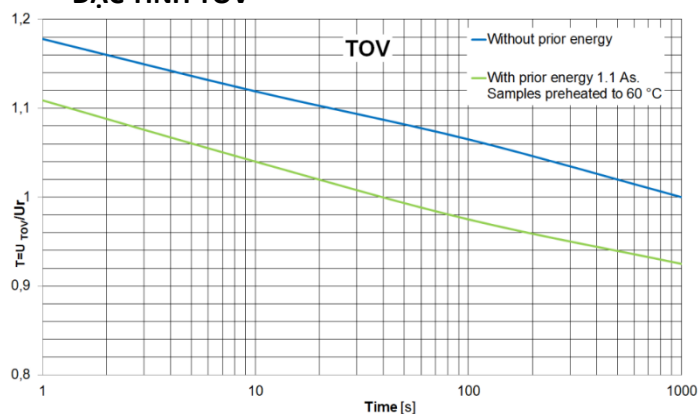
Đặc tính TOV của PROXAR-IN AC
