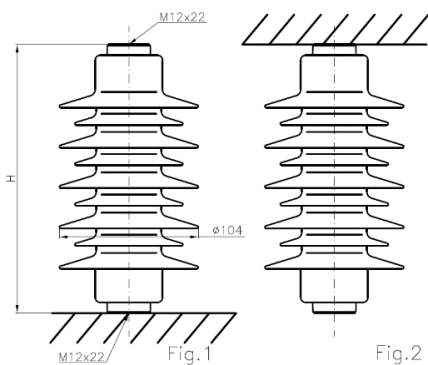
Hình: Thiết bị chống sét PROXAR-IN AC
